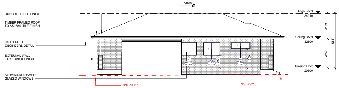
2 Elevation 2 1 : 100
