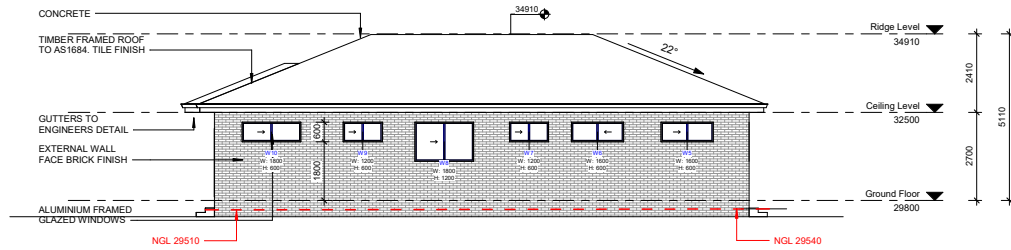
1 Elevation 1. 1 : 100
