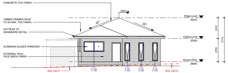
1 Elevation 1 1 : 100
